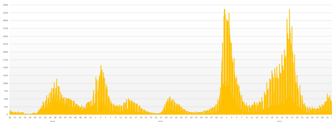
Gráfico 2. Distribución temporal del número de casos confirmados de COVID-19 para personas con edad igual o mayor de 60 años desde el 11 de mayo de 2020. Comunidad de Madrid, datos hasta la semana 43* de 2022.
