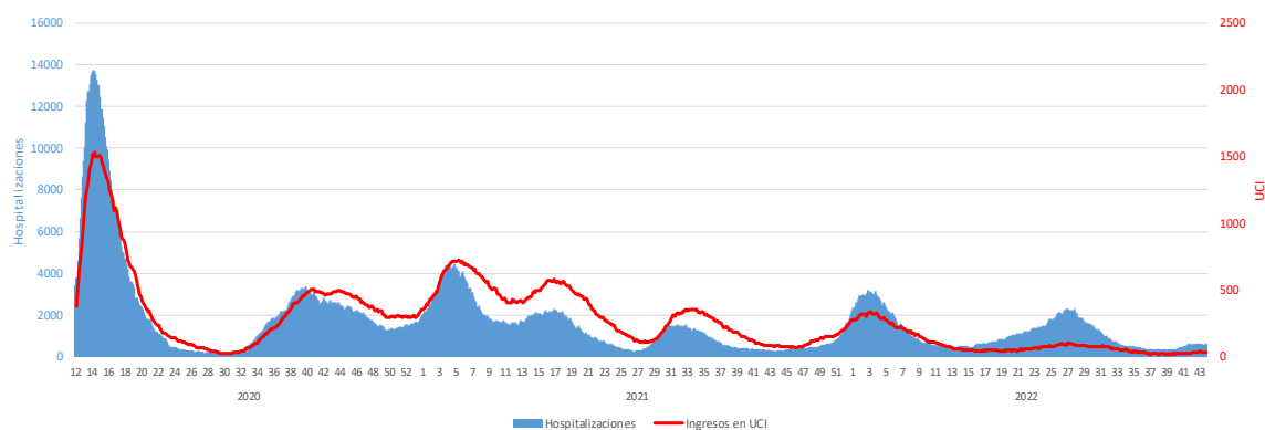
Gráfico 5. Distribución temporal diaria del número de casos que permanecen hospitalizados y en unidades de cuidados intensivos. Comunidad de Madrid, desde el inicio de la pandemia hasta la semana 43 de 2022.
