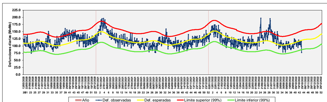
Gráfico 10. Mortalidad diaria, valores observados y esperados, todas las edades. Comunidad de Madrid, datos a partir del 11 de mayo de 2020 hasta la semana 43 de 2022.
