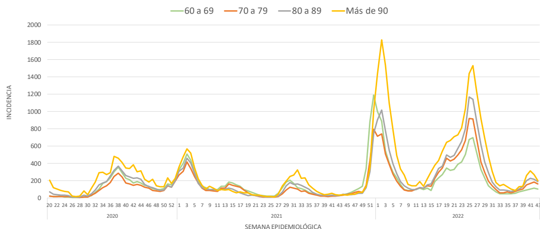
Gráfico 3. Distribución temporal de la incidencia* de los casos confirmados de COVID-19 para personas con edad igual o mayor de 60 años. Comunidad de Madrid, datos hasta la semana 43** de 2022.
